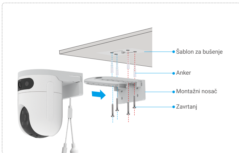
Slika 1. Montaža na plafon
