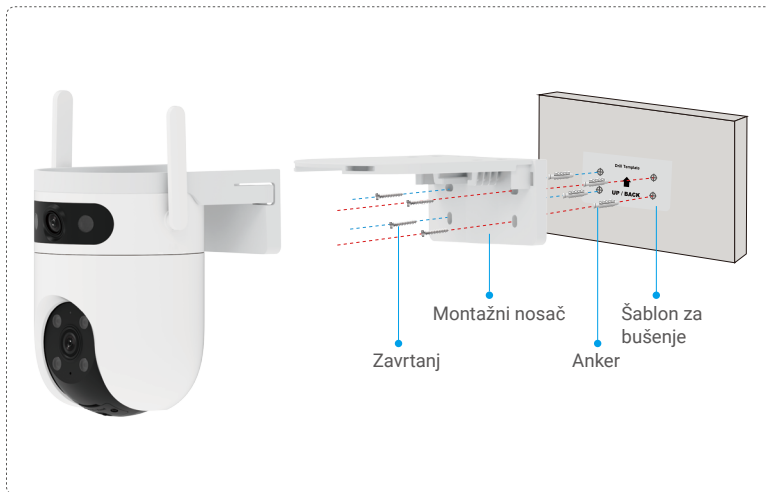
Slika 2. Montaža na zid
